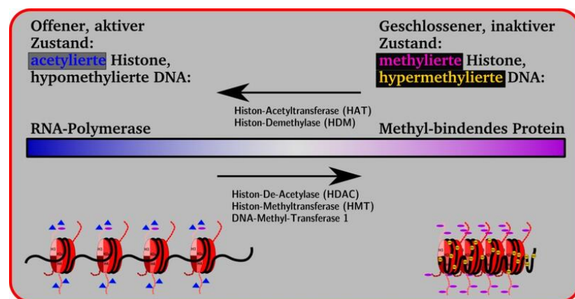
Abbildung 2: Schematische Darstellung der Histon-Methylierung und -Acetylierung sowie der Methylierung von DNA. Die Pfeile symbolisieren jene speziellen Proteine, die für das Anbringen und Entfernen der chemischen Veränderungen zuständig sind. Bild: Bernhard Kleine, CC BY-SA 3.0 DE, via Wikimedia Commons
